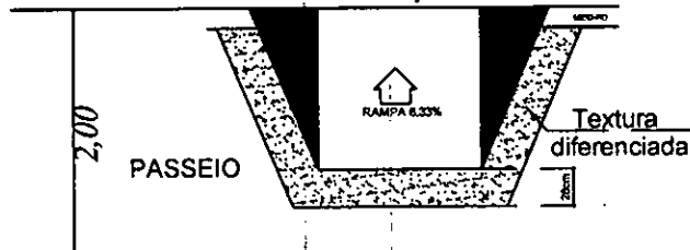
PLANTA DEMARCAÇÃO
