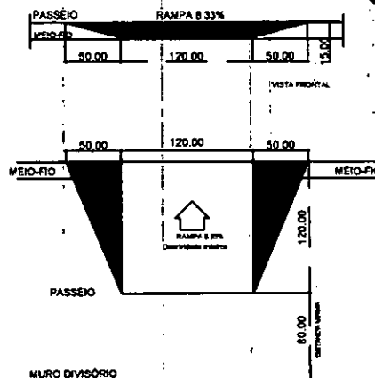
PLANTA BAIXA
