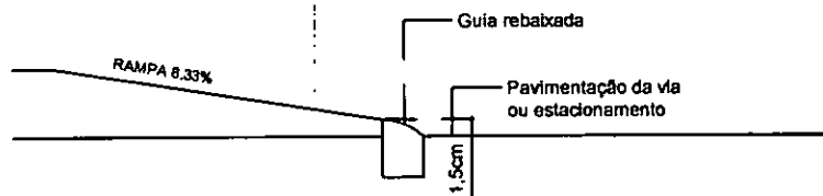
DETALHE leito carroçável
