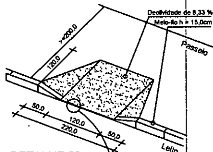
DETALHE 02
